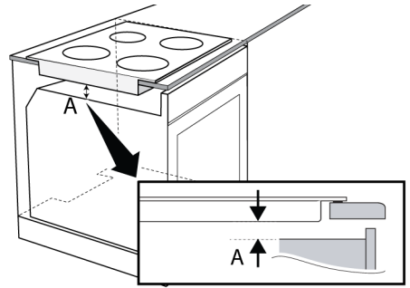
A мин 15 мм
